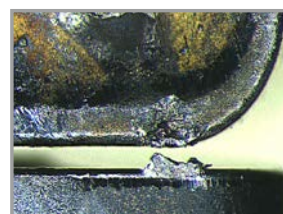
Inserto rivestito CVD convenzionale
